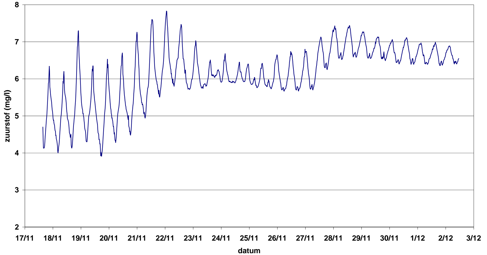
160800 SCHELDE te Kruibeke - stroomafwaarts Rupel zuurstofgehalte (mg/L) - periode 17/11 tem 2/12/2008
